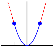
(d) huber, \kappa = 1
